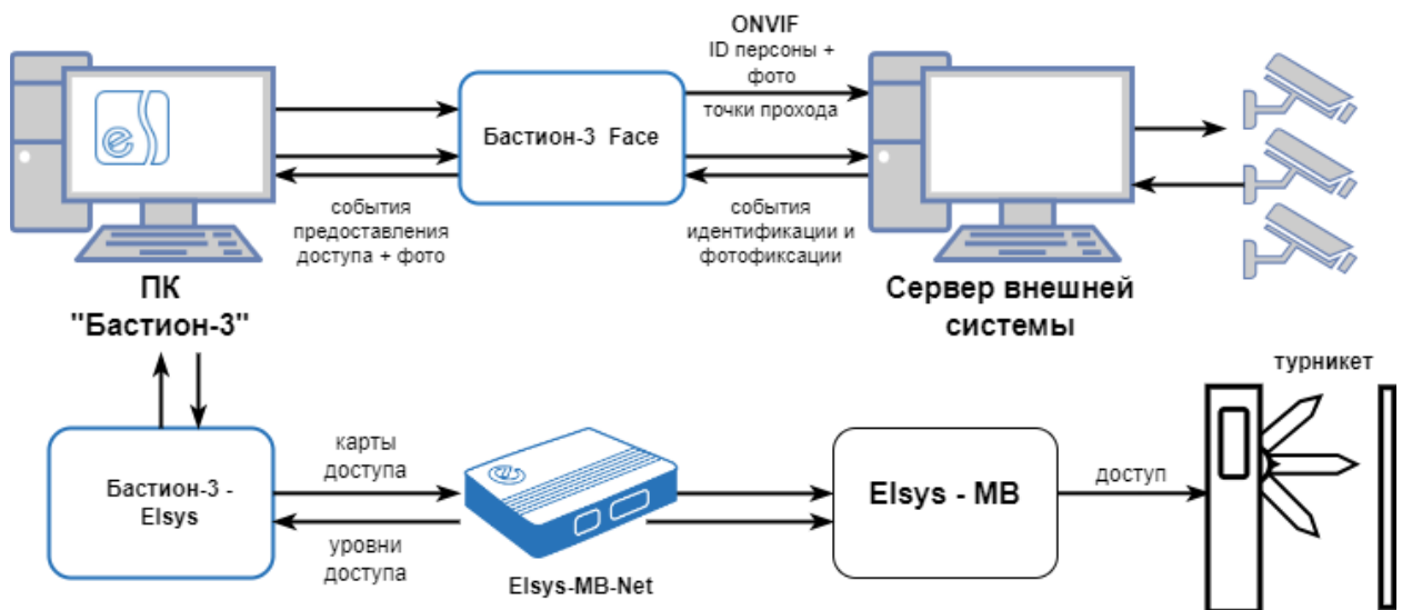
Рис. 9. Работа системы в режиме идентификации
