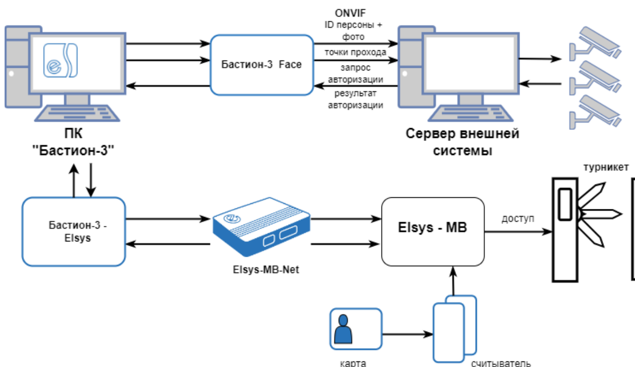
Рис. 8. Работа системы в режиме двухфакторной аутентификации
